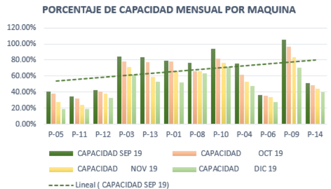
Figura 32. Gráfico de aprovechamiento de equipos de producción. Fuente: Elaboración propia
