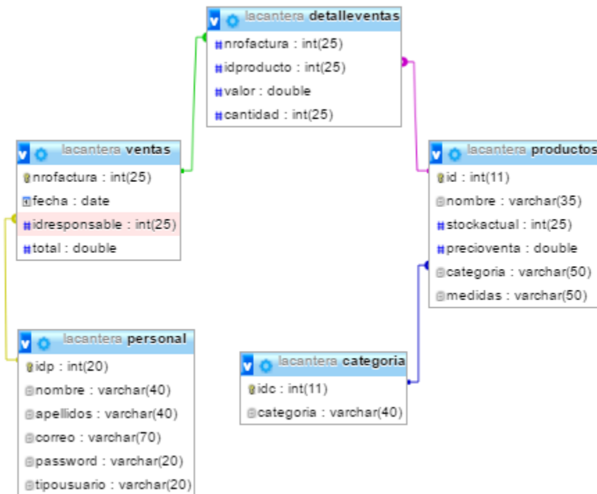
Ilustración 29 Diseño de la base de datos
