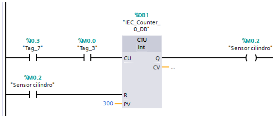
Figura 3.1.7. Contador de enclaves de tapas.
