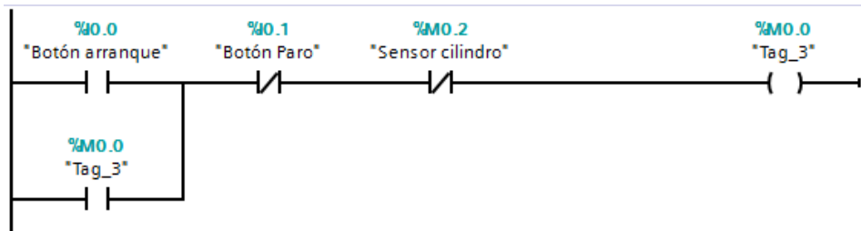
Figura 3.1.5. Línea de arranque y paro
