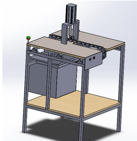
Figura 3.1.13 Diseño 3D de la máquina de enclave.
